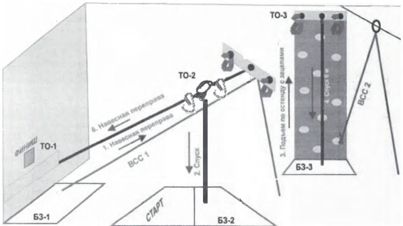
Схема дистанции. Расположение ТЮ, ВСС и БЗ.
